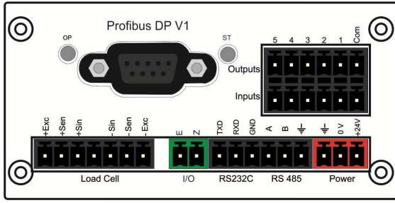
BX11 PB arkadan görünümü
