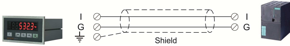
Şekil 4.10 - BX11 AN Akım çıkış bağlantısı
