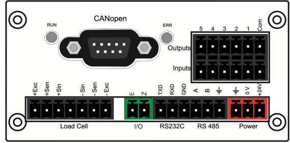
BX11 C0 arkadan görünümü
