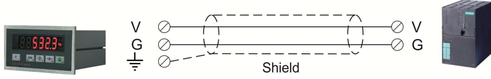
Şekil 4.9 – BX11 AN Gerilim çıkış bağlantısı
