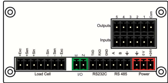
BX11 & BX11 MB arkadan görünümü
