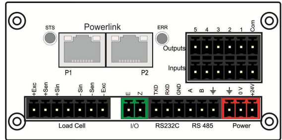
BX11 PL arkadan görünümü
